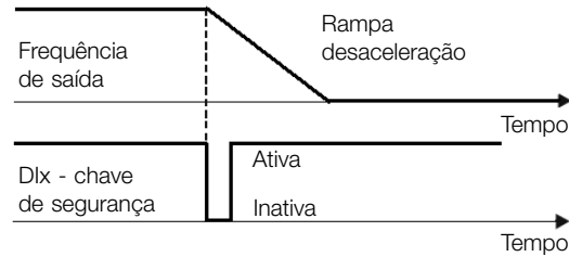
Figura 9.17: Exemplo da função Emergência
