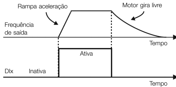
Figura 9.7: Exemplo da função Habilita Geral
