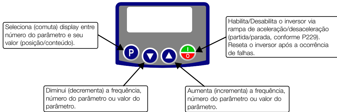
Figura 4.1: Teclas da HMI
