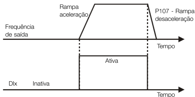
Figura 9.8: Exemplo da função Parada Rápida
