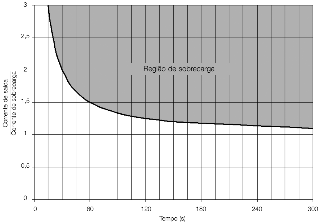
Figura 10.2: Atuação da sobrecarga do motor
