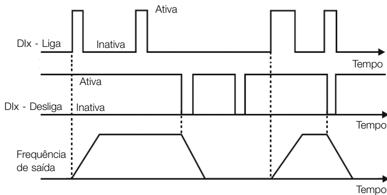
Figura 9.10: Exemplo da função Liga/Desliga
