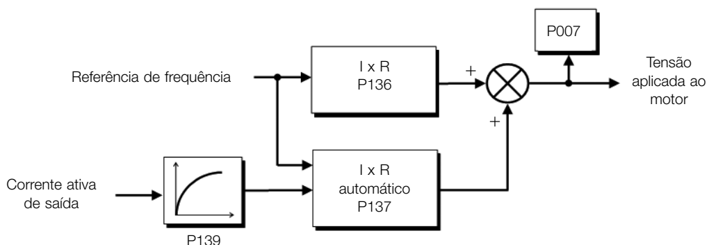
Figura 8.17: Blocodiagrama do boost de torque automático
