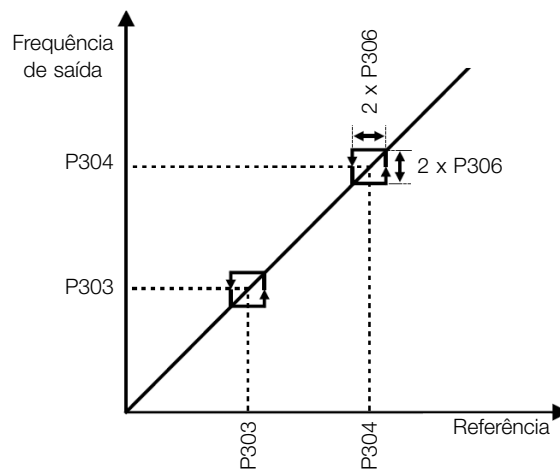
Figura 8.11: Atuação da frequência evitada
