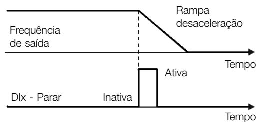
Figura 9.16: Exemplo da função Parar
