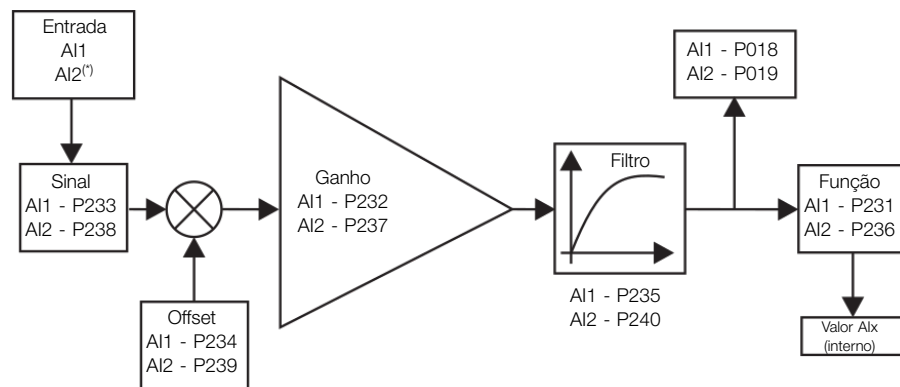
Figura 9.1: Diagrama de blocos das entradas analógicas (Alx)
