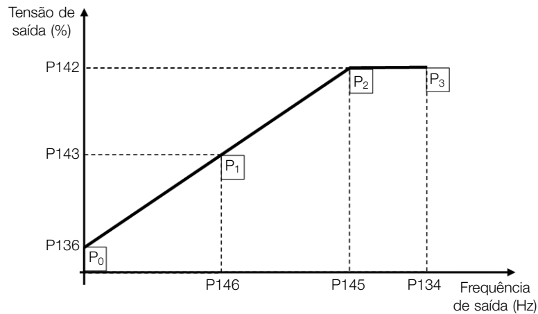
Figura 8.13: Curva V/f
