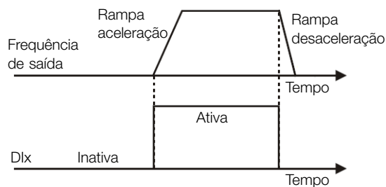
Figura 9.6: Exemplo da função Gira/Para
