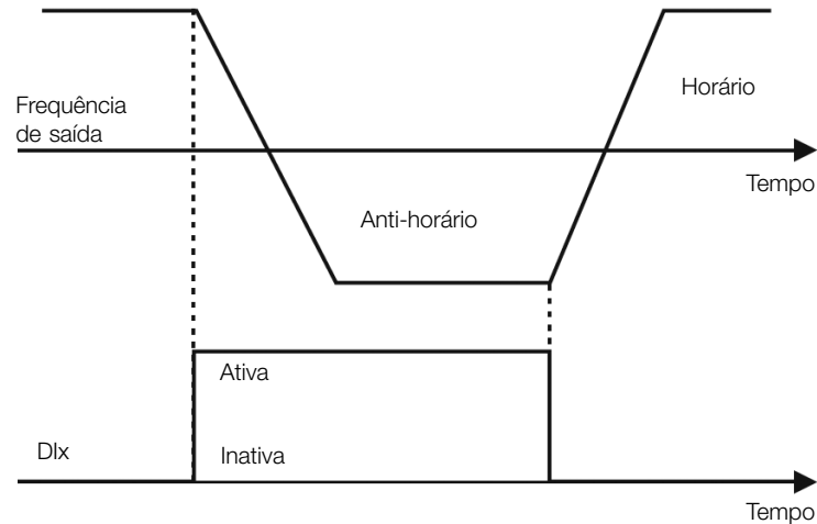
Figura 9.11: Exemplo da função Sentido de Giro
