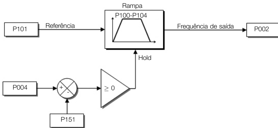
Figura 8.3: Blocodiagrama da limitação da tensão do Link DC
